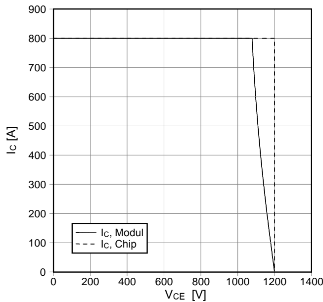
Sicherer Rückwärts-Arbeitsbereich IGBT-Wr. (RBSOA) reverse bias safe operating area IGBT-inv. (RBSOA) I_C = f(V_{CE}) V_{GE} = \pm 15\text{ V} , R_{Goff} = 2,2\ \Omega , T_{vj} = 125^\circ\text{C}
