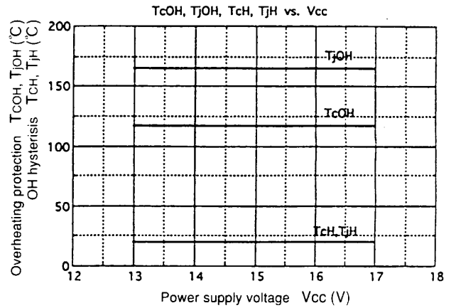
過熱保護動作温度—電源電圧特性 Overheating characteristics T_{COH} , T_{OH} , T_{CH} , T_{JH} vs. V_{CC}
